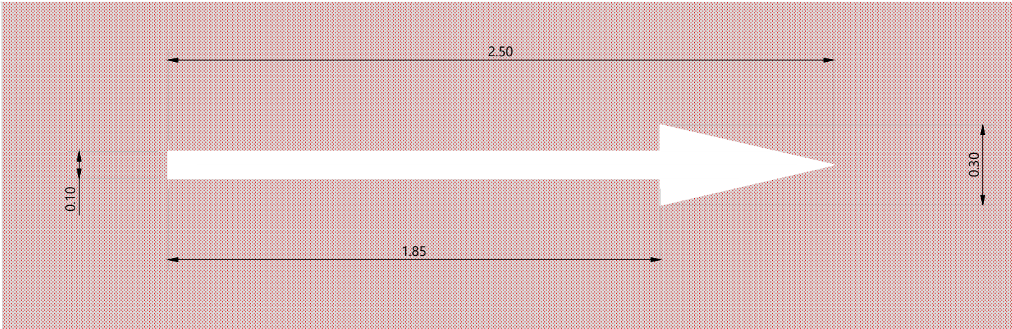
AFMETINGEN PULMARKERING FIETSPAD Schaal 1:20
