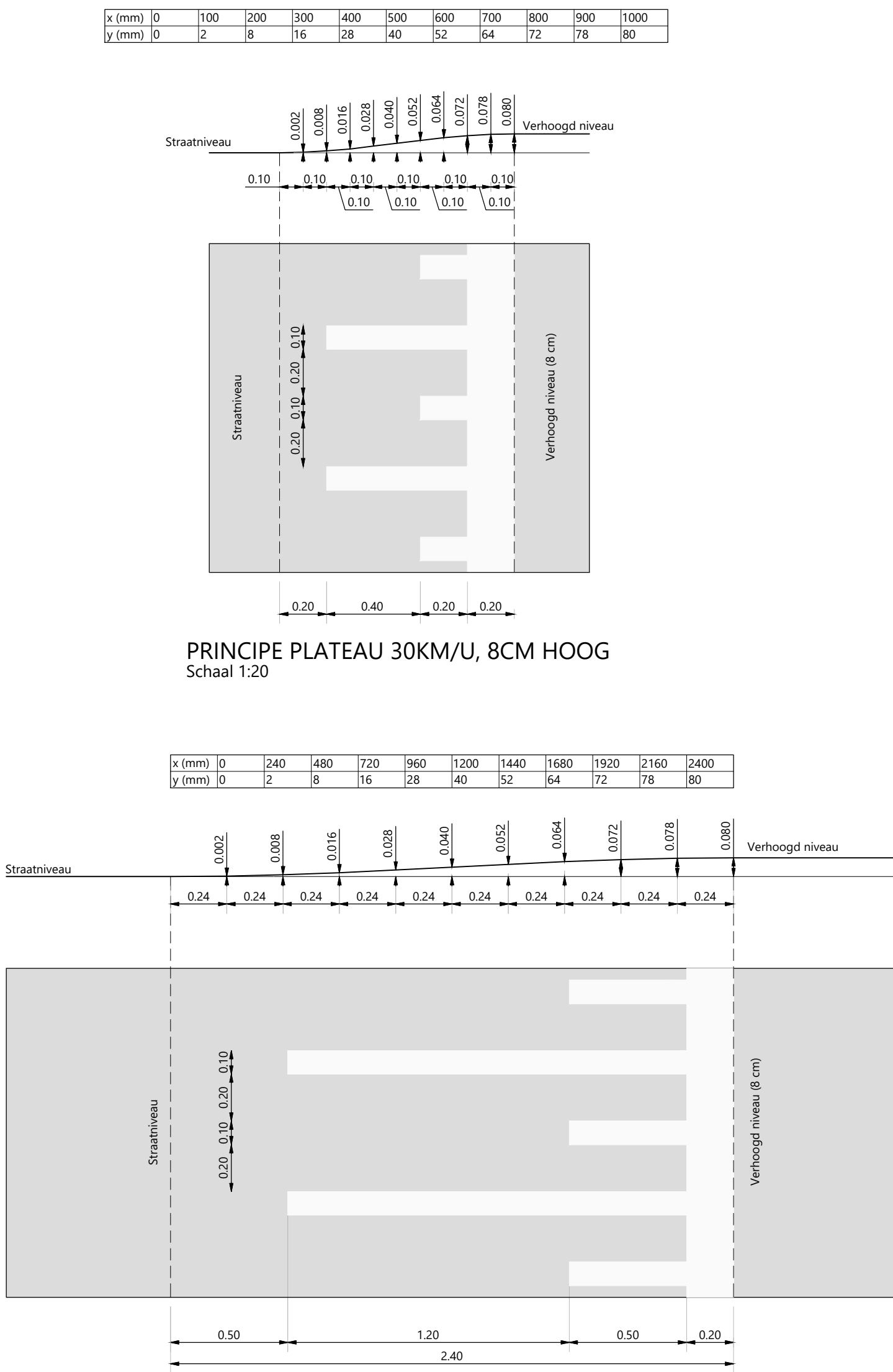
PRINCIPE PLATEAU 30KM/U, 8CM HOOG Schaal 1:20 PRINCIPE SINUSPLATEAUS 8cm 50 km/u Schaal 1:20
