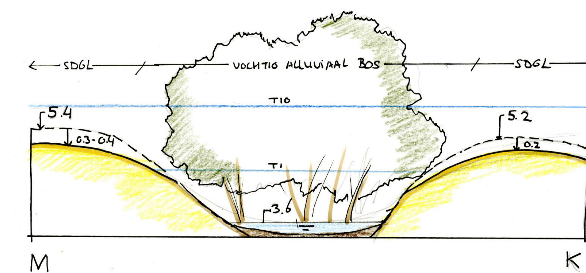
Principeprofiel
