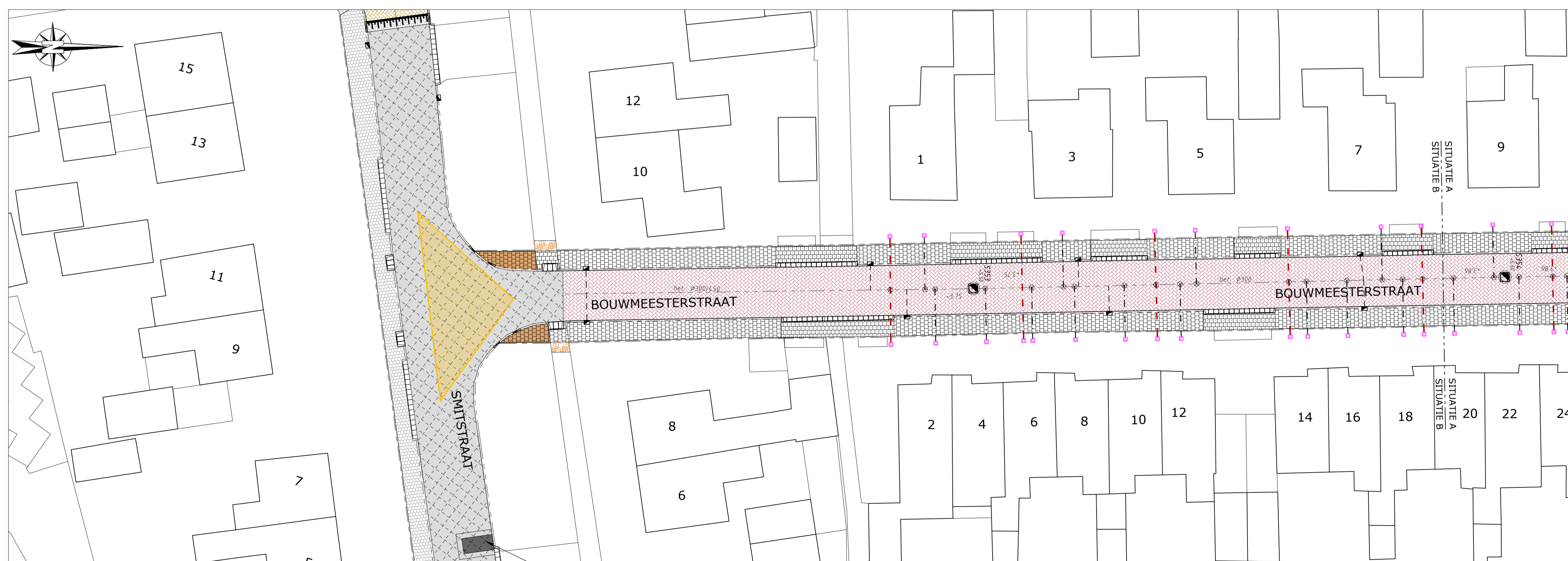
SITUATIE B-B
