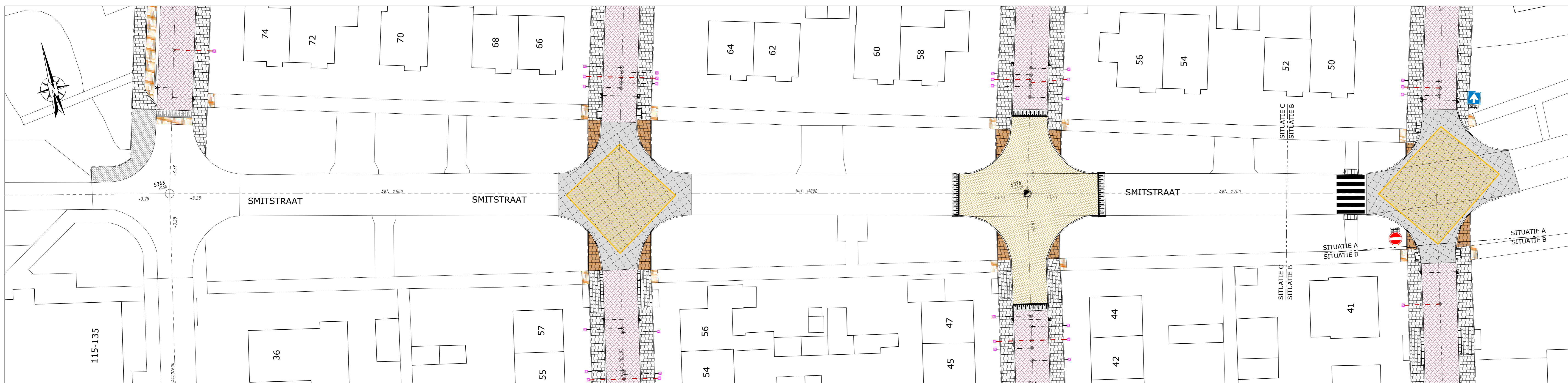
SITUATIE C-C
