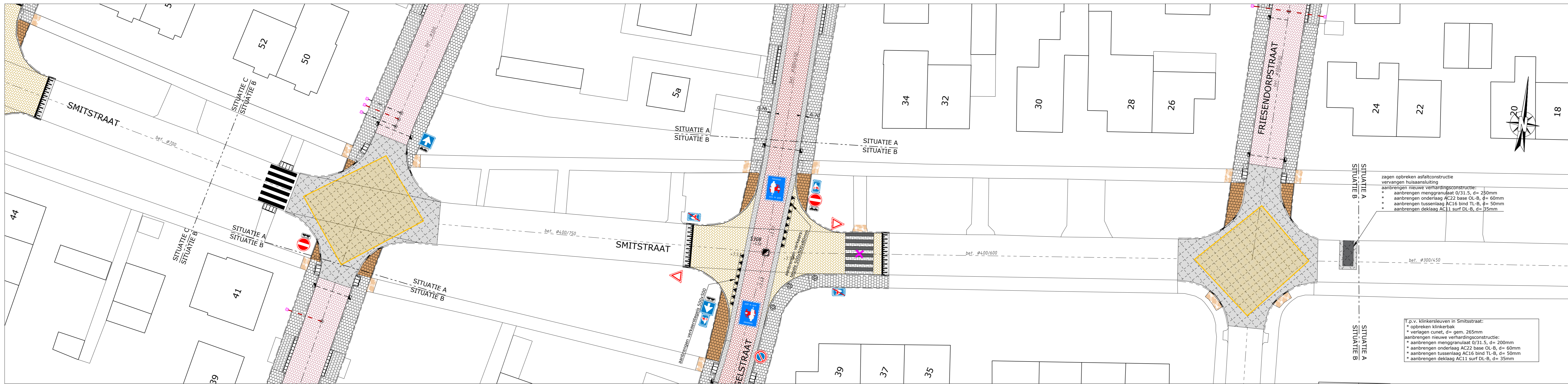
SITUATIE B-B
