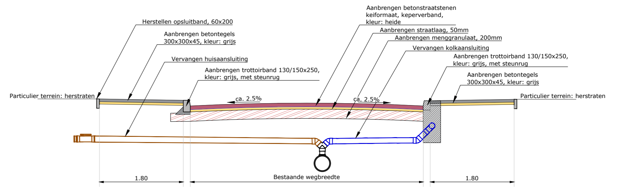
PRINCIPE DOORSNEDE RIJBAAN
