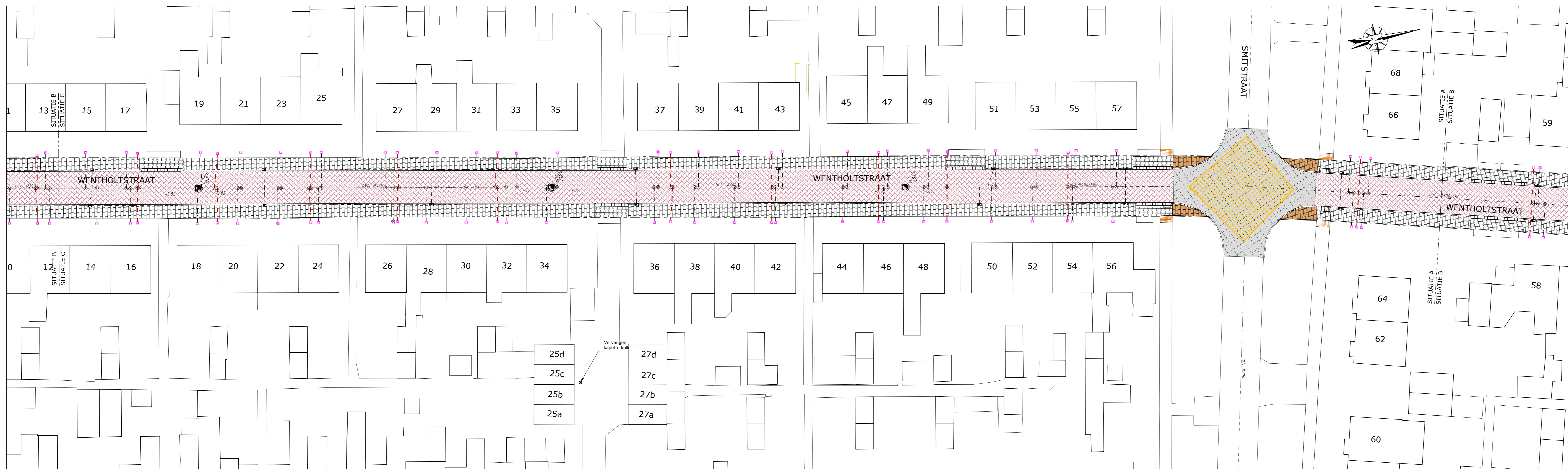
SITUATIE B-B
