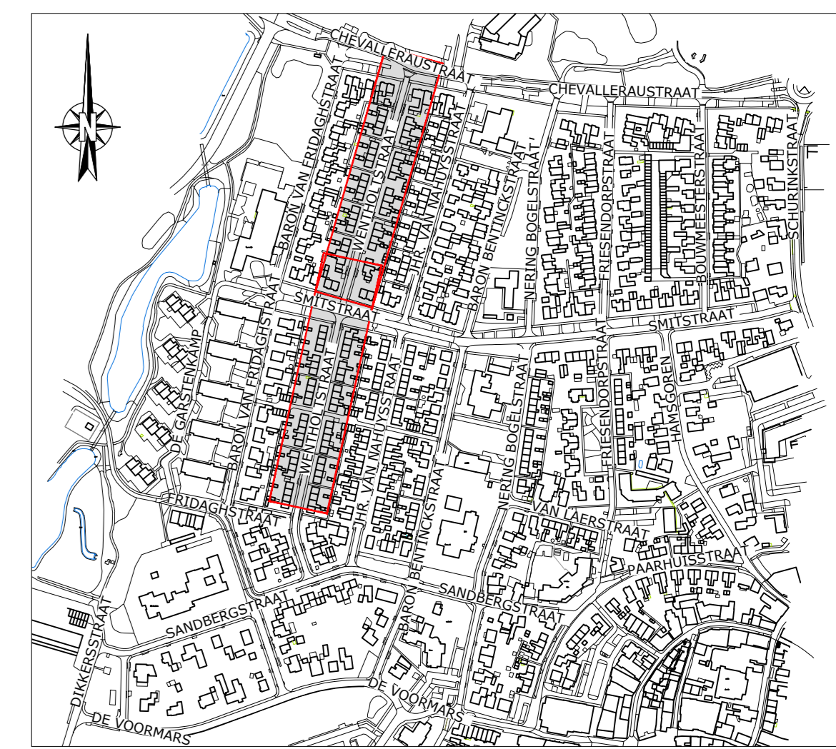
SITUATIE OVERZICHT
