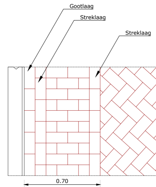
DETAIL RABATSTROOK FIETSSTRAAT
