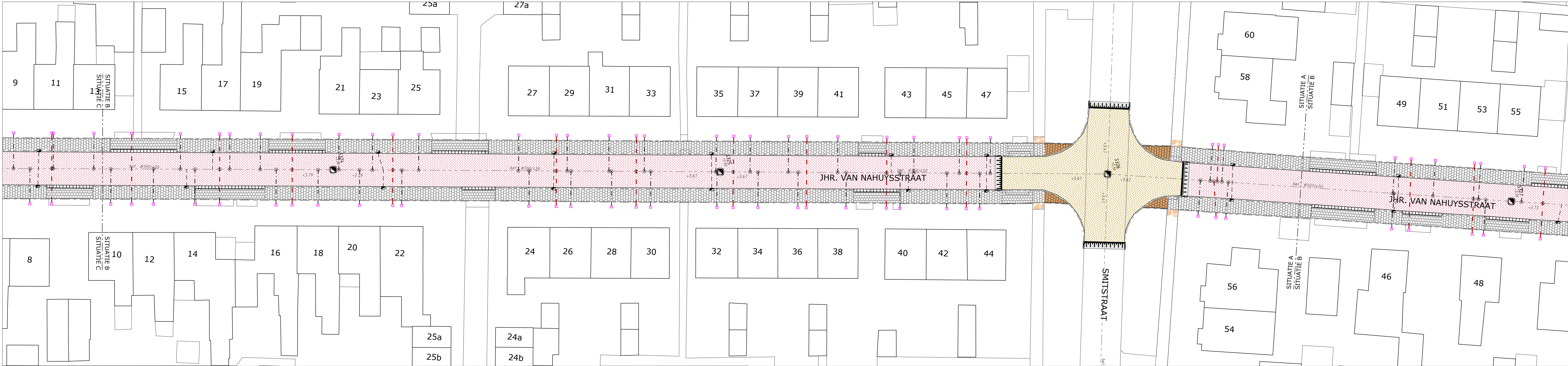
SITUATIE B-B
