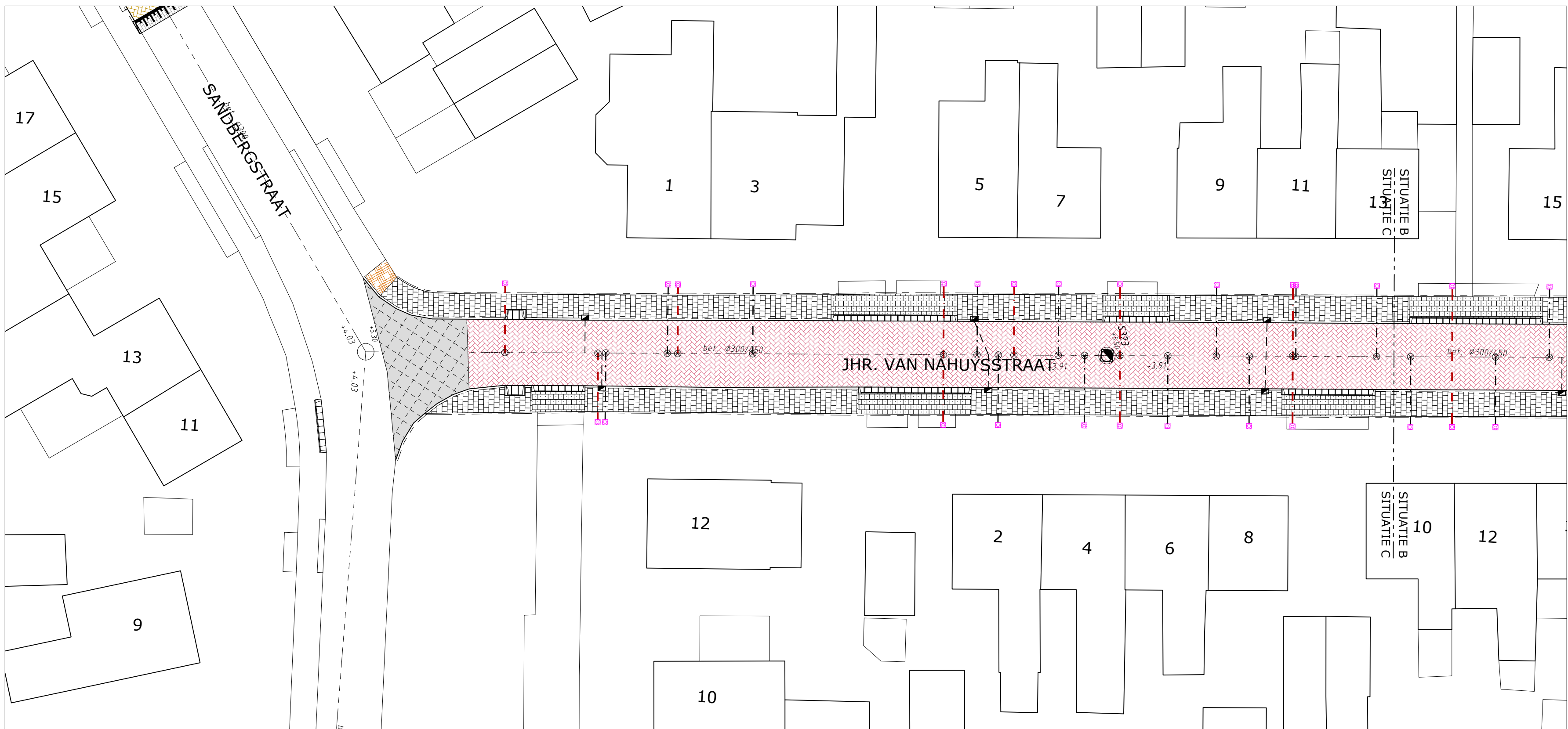
SITUATIE C-C
