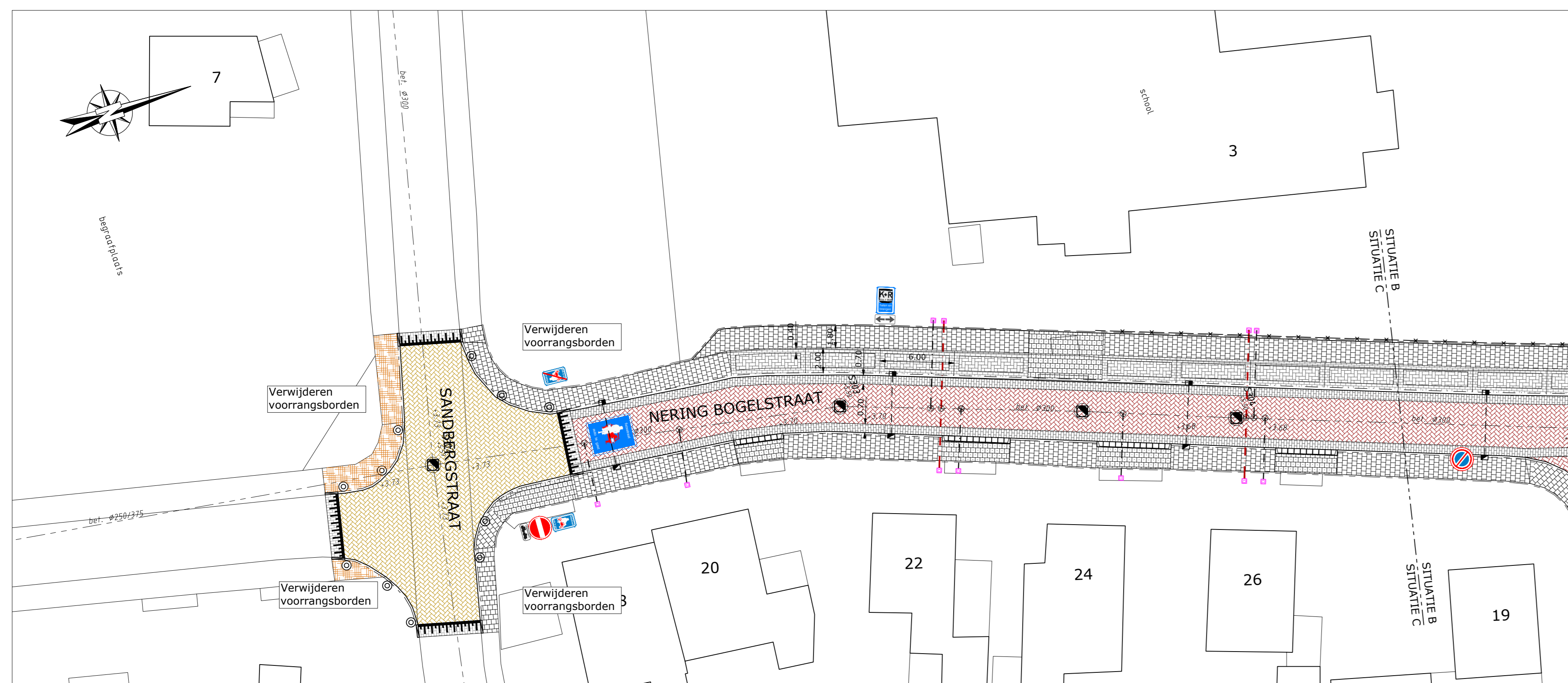
SITUATIE C-C
