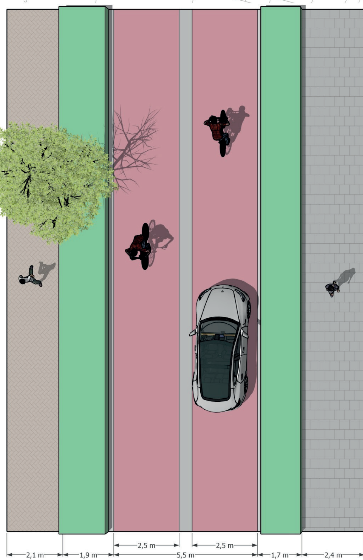
dwarsprofiel
